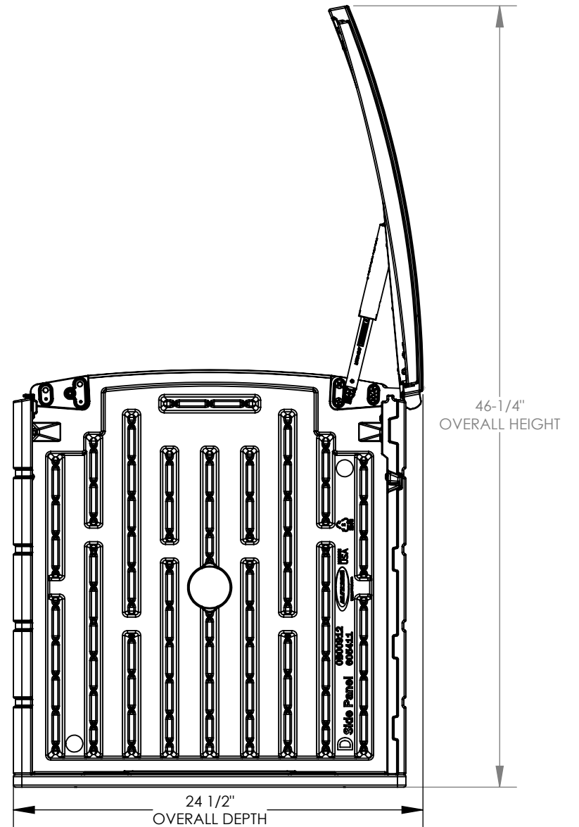
SECTION B-B SCALE 1 : 8
