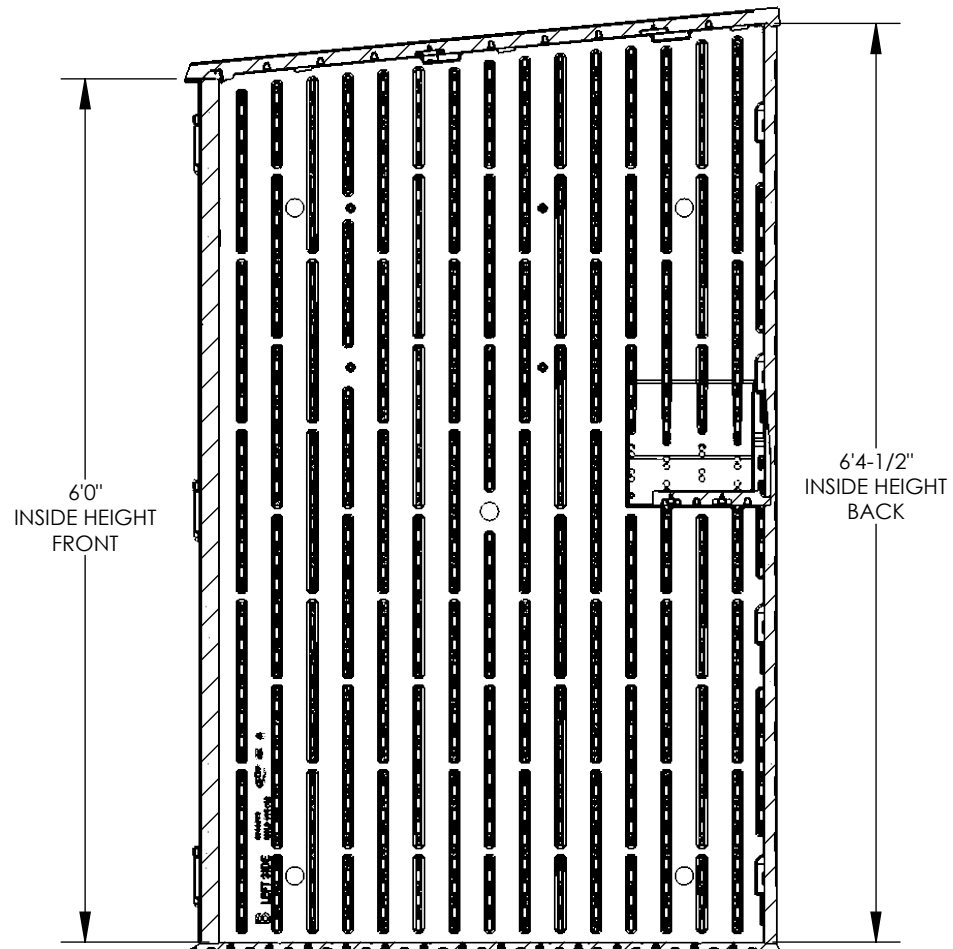
SECTION B-B SCALE 1 : 16
